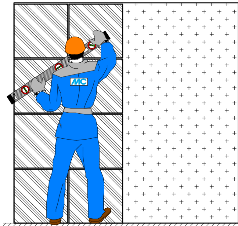
Рис.30. Последовательность работ, где: 1 – проверка ровности основания контрольной рейкой; 2, 3 – приготовление грунтовки; 4 – нанесение грунтовки на цементную штукатурку; 5 – приготовление клеевой смеси; 6, 7 – нанесение клеевой смеси на основание (захватками); 8, 9 – приклеивание керамогранитной плитки на стену (захватками); 10 – проверка облицовки при помощи уровня. ПРИМЕЧАНИЕ к рис 30.: на этапах 6-9 указано проведение работ в направлении снизу вверх, но при использовании клеев, в маркировке которых присутствует буква «Т», возможно выполнение работ в направлении сверху вниз.
