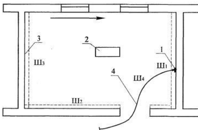
Рис. 25. Схема организации рабочего места звена № 1
